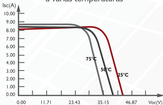
Curva I-V de módulo SAYA-330-72 a varias temperaturas
