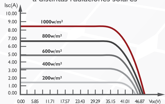
Curva I-V de módulo SAYA-P330-72 a distintas radiaciones solares
