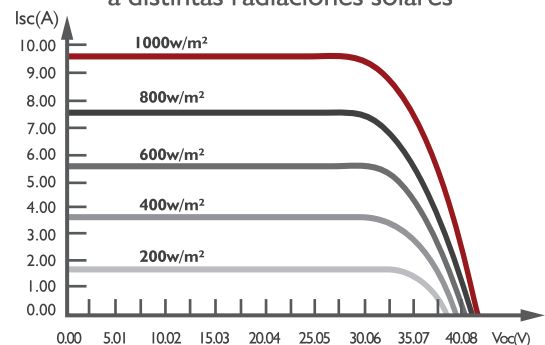
Curva I-V de módulo SAYA-325M-60 a distintas radiaciones solares
