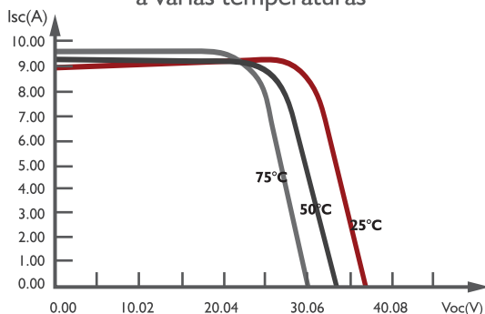
Curva I-V de módulo SAYA-325M-60 a varias temperaturas
