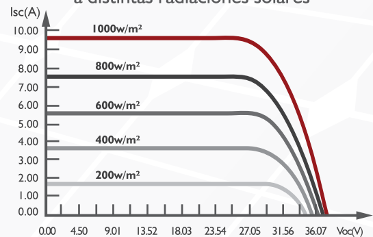
Curva I-V de módulo SAYA-290M-54 a distintas radiaciones solares
