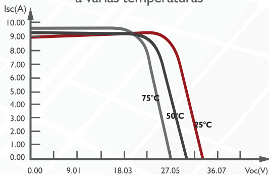
Curva I-V de módulo SAYA-290M-54 a varias temperaturas
