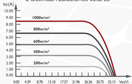
Curva I-V de módulo SAYA-P250-54 a distintas radiaciones solares
