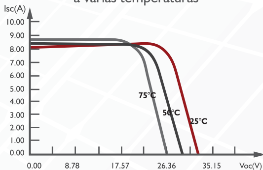
Curva I-V de módulo SAYA-P250-54 a varias temperaturas
