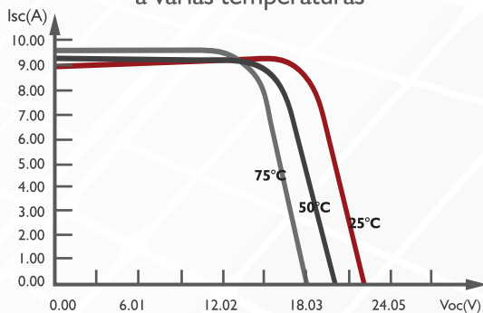
Curva I-V de módulo SAYA-195M-36 a varias temperaturas
