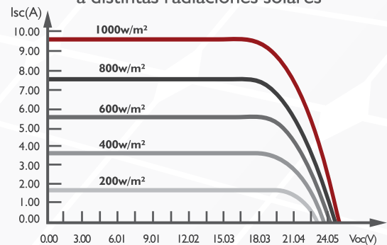
Curva I-V de módulo SAYA-195M-36 a distintas radiaciones solares
