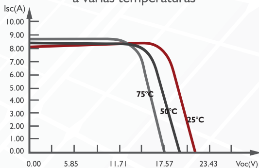
Curva I-V de módulo SAYA-PI 170-36 a varias temperaturas
