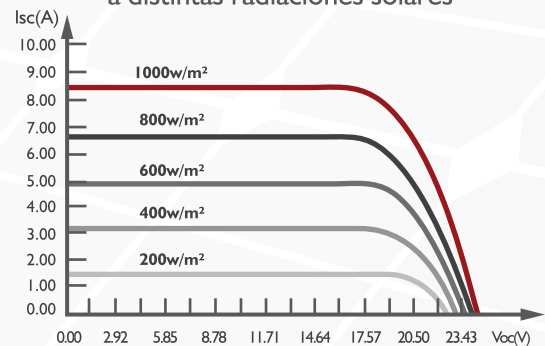
Curva I-V de módulo SAYA-PI 170-36 a distintas radiaciones solares
