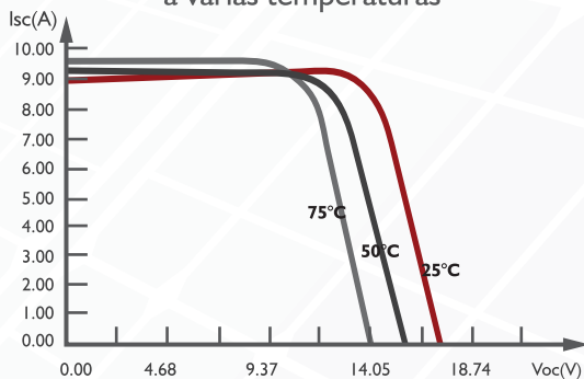
Curva I-V de módulo SAYA-150M-28 a varias temperaturas
