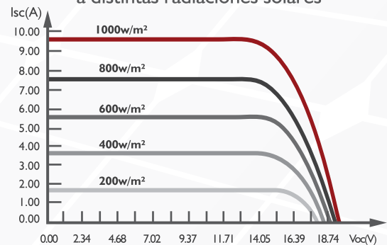
Curva I-V de módulo SAYA-150M-28 a distintas radiaciones solares
